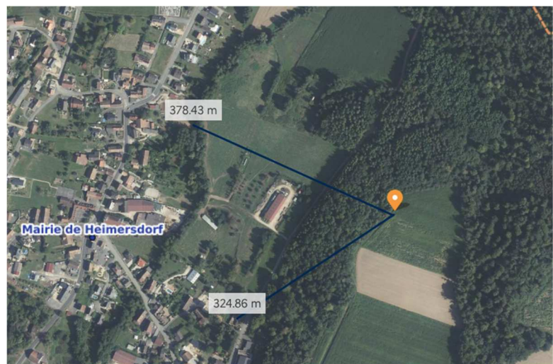
Implantation de l'antenne-relais
